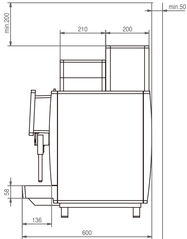
天板開口位置
