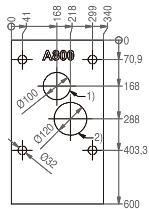
天板開口位置
